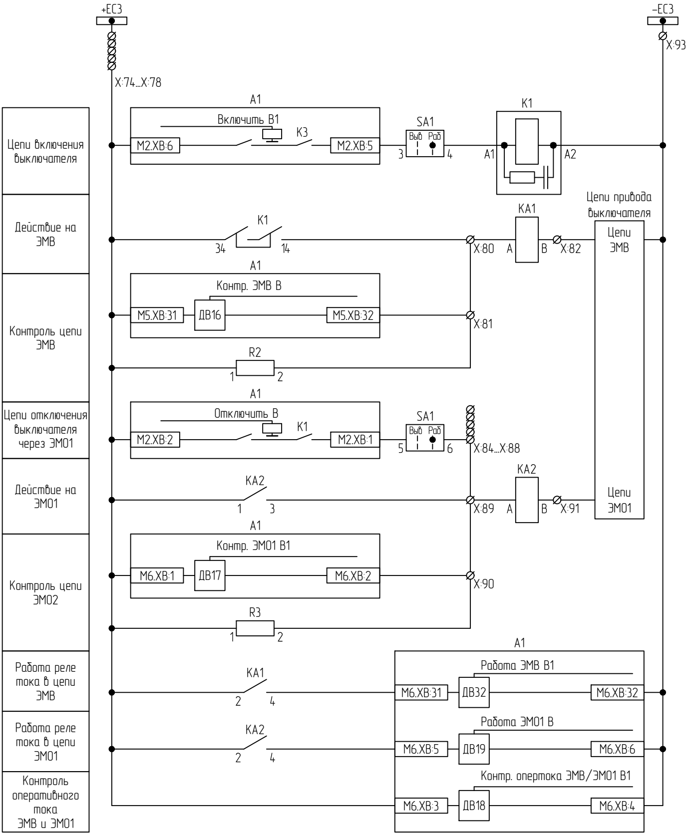
Цепи ЭМВ и ЭМ01
